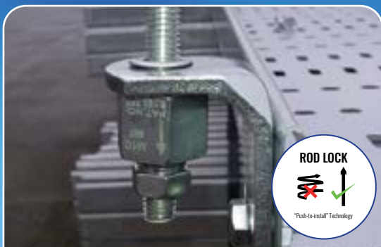
ROD LOCK
